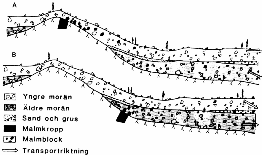
Fig. 1. Blockspridningen från två olika malmkroppar. De flesta malmblocken ligger intill malmen. (Efter Hirvas 1981)
