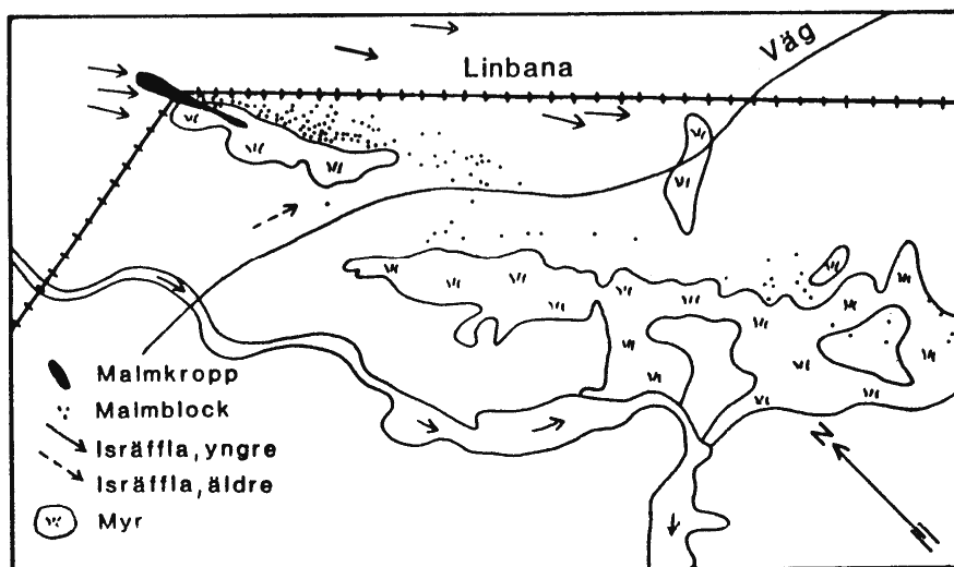
Fig. 2. Rakkejaurmalmen lokaliserades enbart med hjälp av blockkletning (Efter E Grip).
