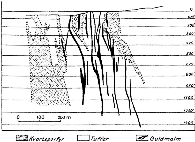
Tvärsektion genom Hollingergruvans system av guldkvartsgångar. Siffrorna, som angiva djupet, äro i fot. Efter A. G. Burrows.
