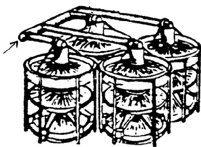
Konapparat för grovavskiljning i ett första steg
