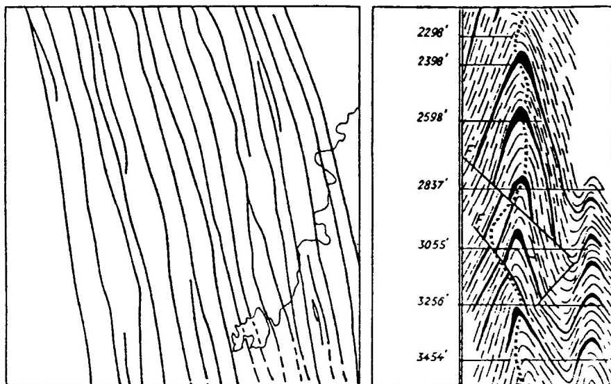
Till vänster karta över de antiktinala axiallinjerna i Bendigo, Australien. Till höger en tvärprofil genom den veckade serien med guldkvartsgångarna i omböjningarna (s.k. sadelgångar). Efter H. Herman.
